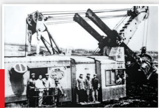
▲1972年9月,灵泉露天煤矿生产时使用的401号电铲。
