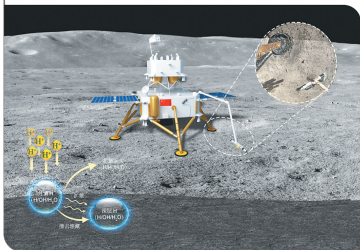
这是太阳风氢的注入、保存与扩散丢失模型图。
